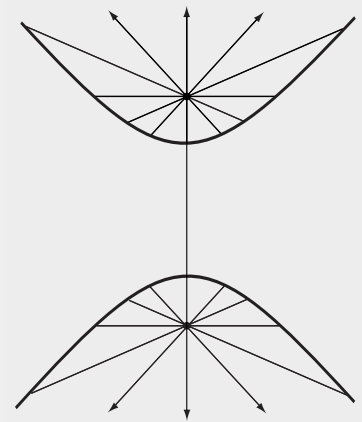
Hyperbola
