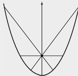
Parabola
